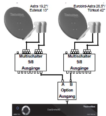
4 satelity (Quattro LNB)
